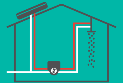
Le SUNPAD est connecté en série avec un chauffe-eau instantané
